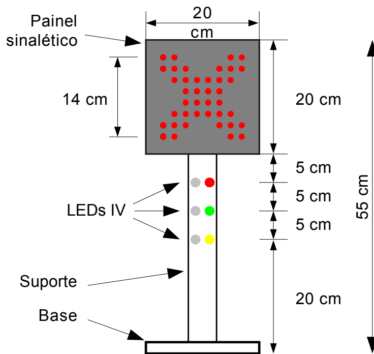
Painel Sinalético - dimensões
