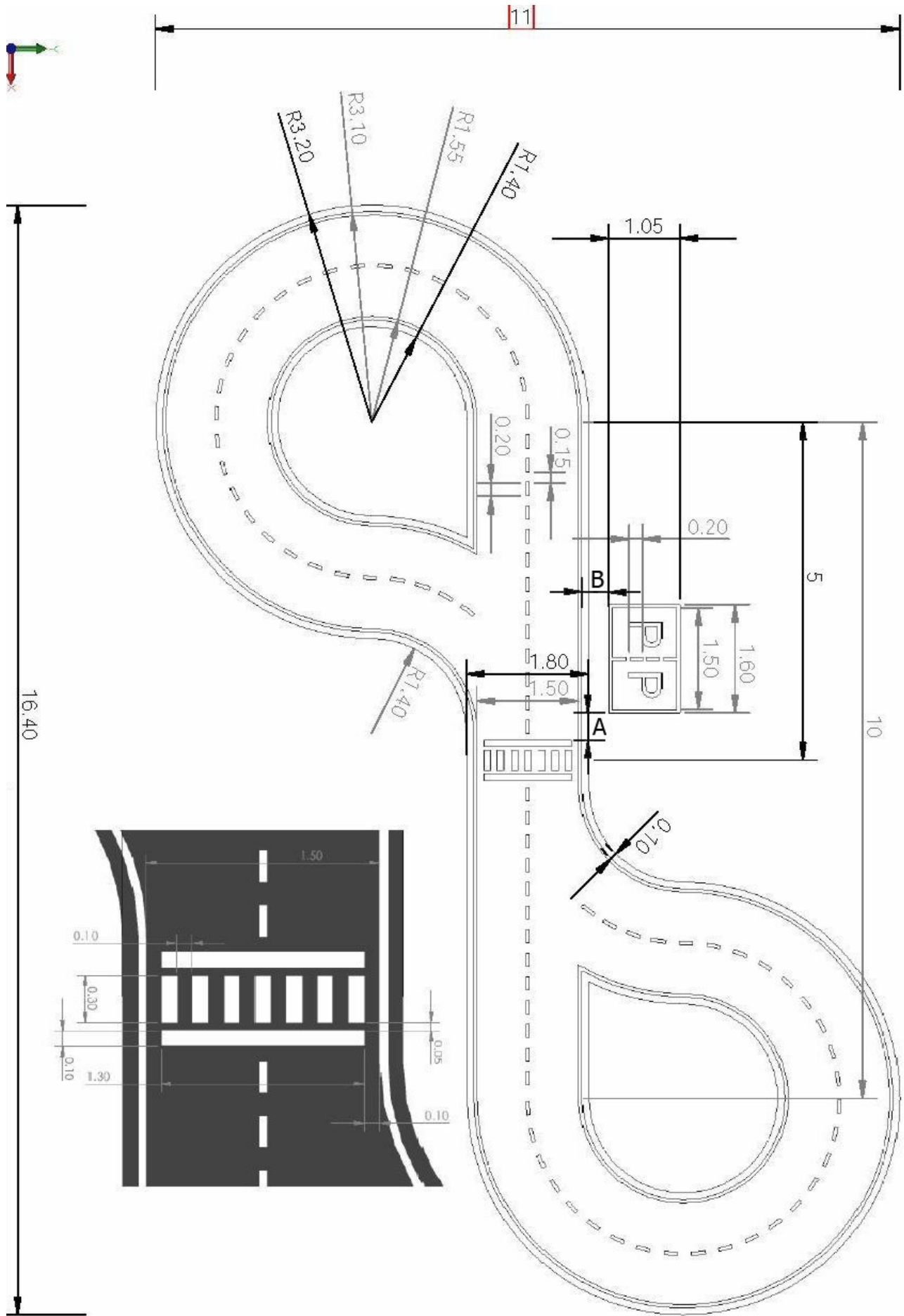
Figura 3 – Dimensões da pista
