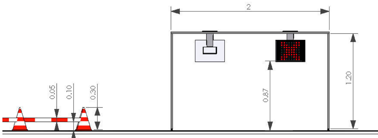
Figura 7 –Painéis sinaléticos e cones da zona de obras - medidas
