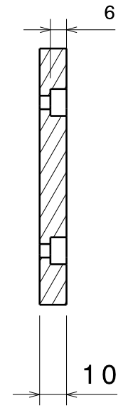
Section view A-A Scale: 1:2
