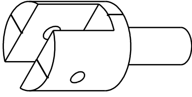
Isometric view Scale: 1:1
