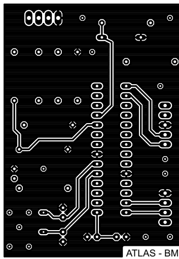
ATLAS - BM
