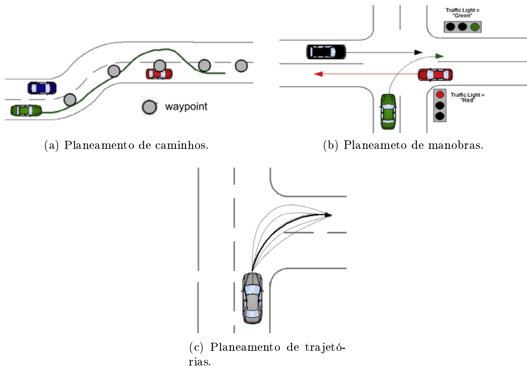
Figura 2.1: Representação dos três diferentes tipos de planejamento/navegação local, (adaptado de Katrakazas et al., (2015)).
