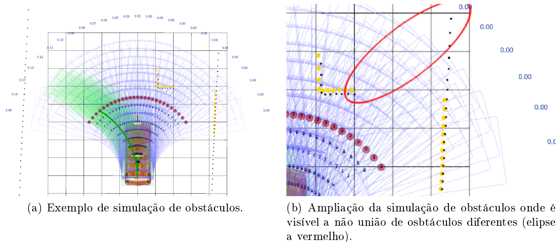
Figura 4.7: Exemplo de detecção de colisões através de inclusões, utilizando a metodologia do WN.
