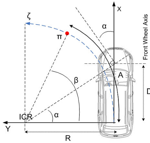
Figura 2.12: Traçado de trajetórias circulares com base num modelo não holonómico de um veículo, (adaptado de Oliveira et al., (2012)).
