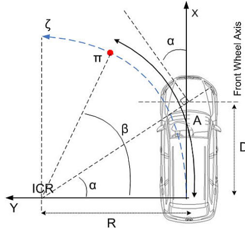
Figura 4.1: Modelo não holonómico de um veículo com direção de Ackermann , (adaptado de Oliveira et al., (2012)).
