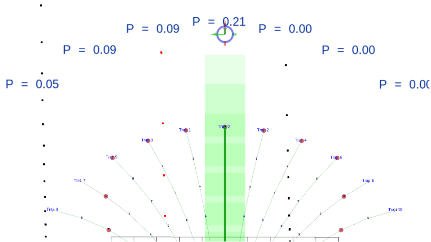
Figura 4.14: Exemplo da afetação da pontuação das trajetórias à esquerda, que interceptam a linha central (pontos a vermelho), pelo parâmetro CL.
