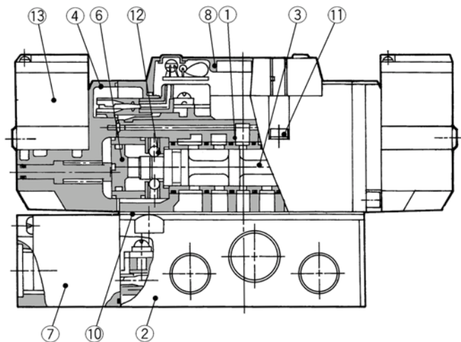
Centro cerrado de 3 posiciones/centro a escape/centro a presión
