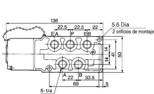
Conexión inferior
