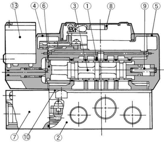
Centro cerrado de 3 posiciones/centro a escape/centro a presión
